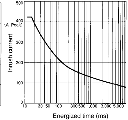
G3PB-235B-VD G3PB-245B-VD
