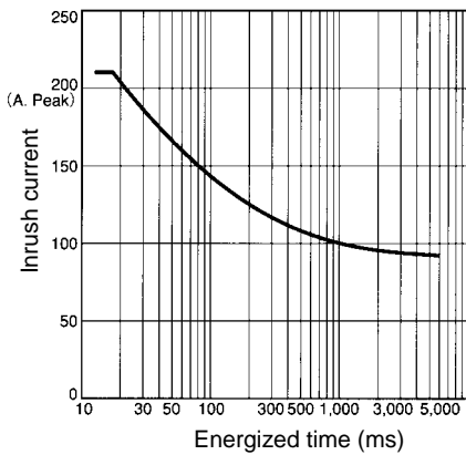
G3PB-225B-VD
