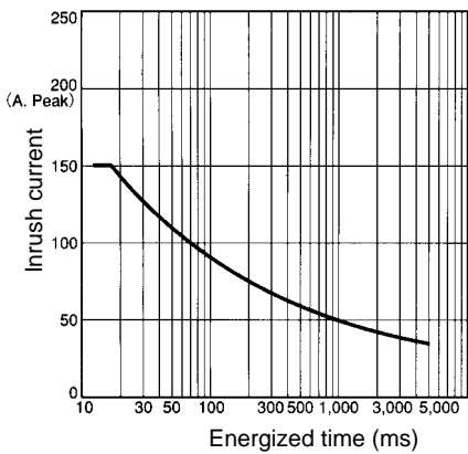
G3PB-215B-VD
