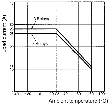
G3PB-235B-VD
